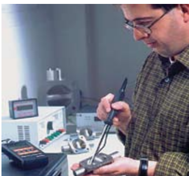
对不锈钢阀体进行铁素体测试。
